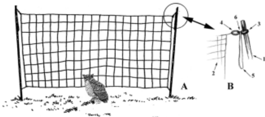
Рис. 29. Опадная сеть и ее крепежный механизм: 1 - колышек, 2 - сеть, 3-4 - крепежные кольца, 5 - шнур, связывающий крепежные кольца, 6 - сторожевая перемычка из резинки.
